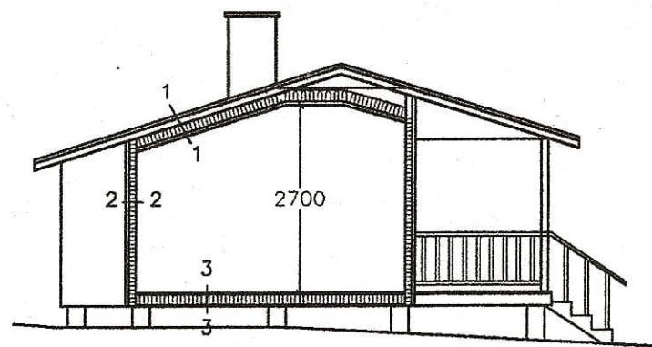
LEIKKAUS A-A 1:100
