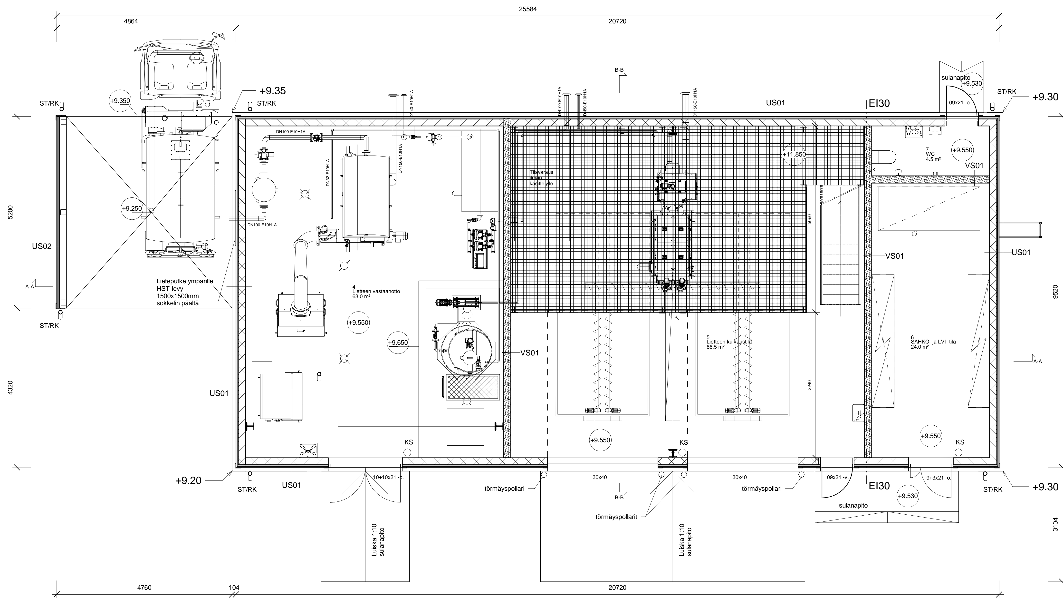
Pohjapiirustus 1. kerros +9.550 1 : 50
